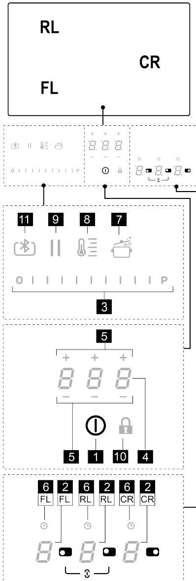
Pannello di controllo mod.603P
