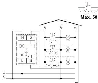
3 huzalos bekötés
