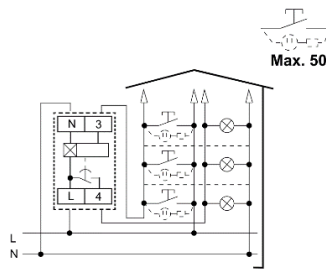
4 huzalos bekötés
